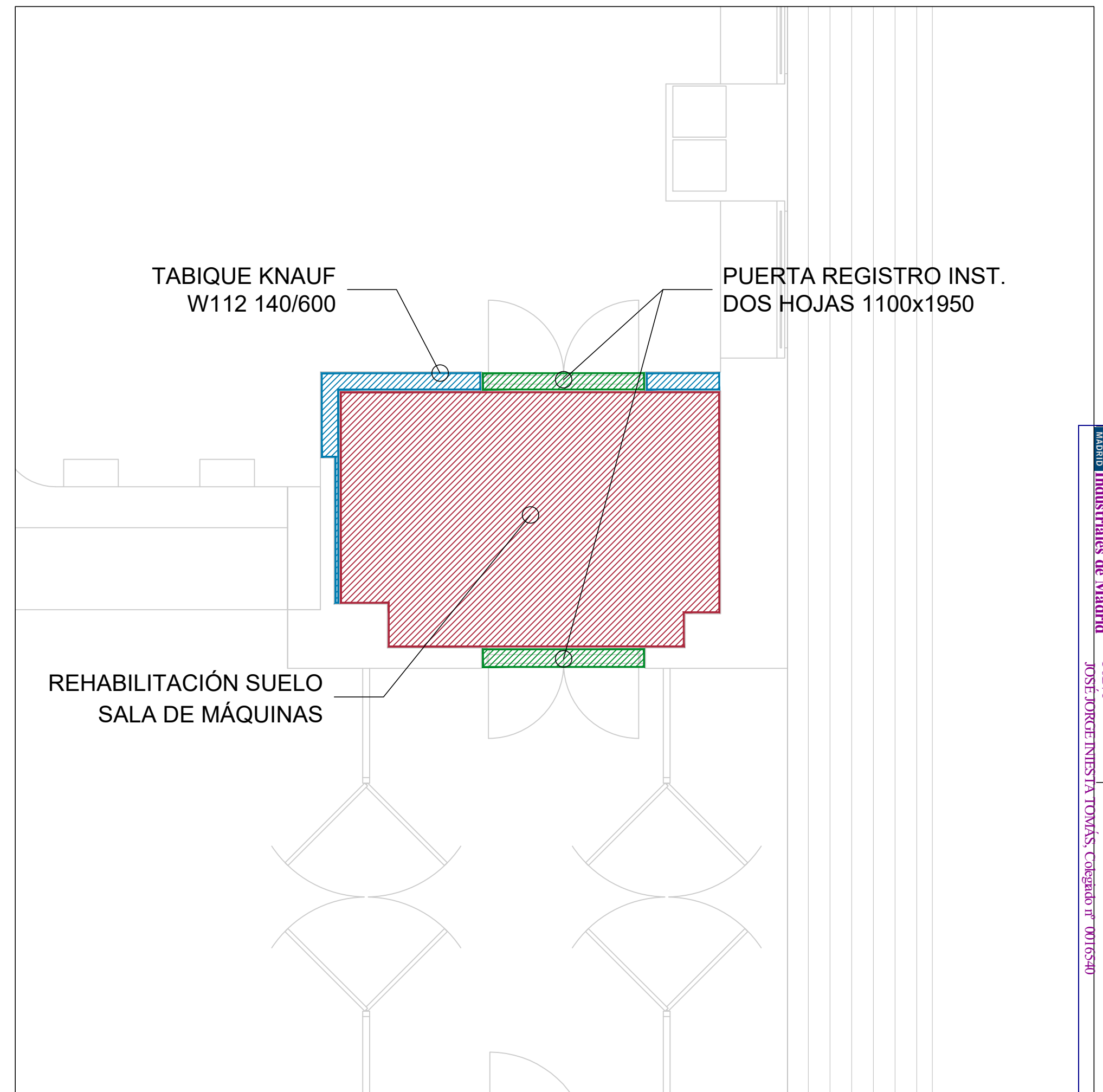
REFORMA SALA MÁQUINAS (ZONA I)
