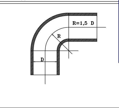
DETALLE (c) : RADIO TÍPICO DE CONDUCTOS
