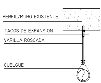
DETALLE 2:
