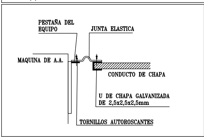
DETALLE (a) : SUBJECCION DE CONDUCTOS
