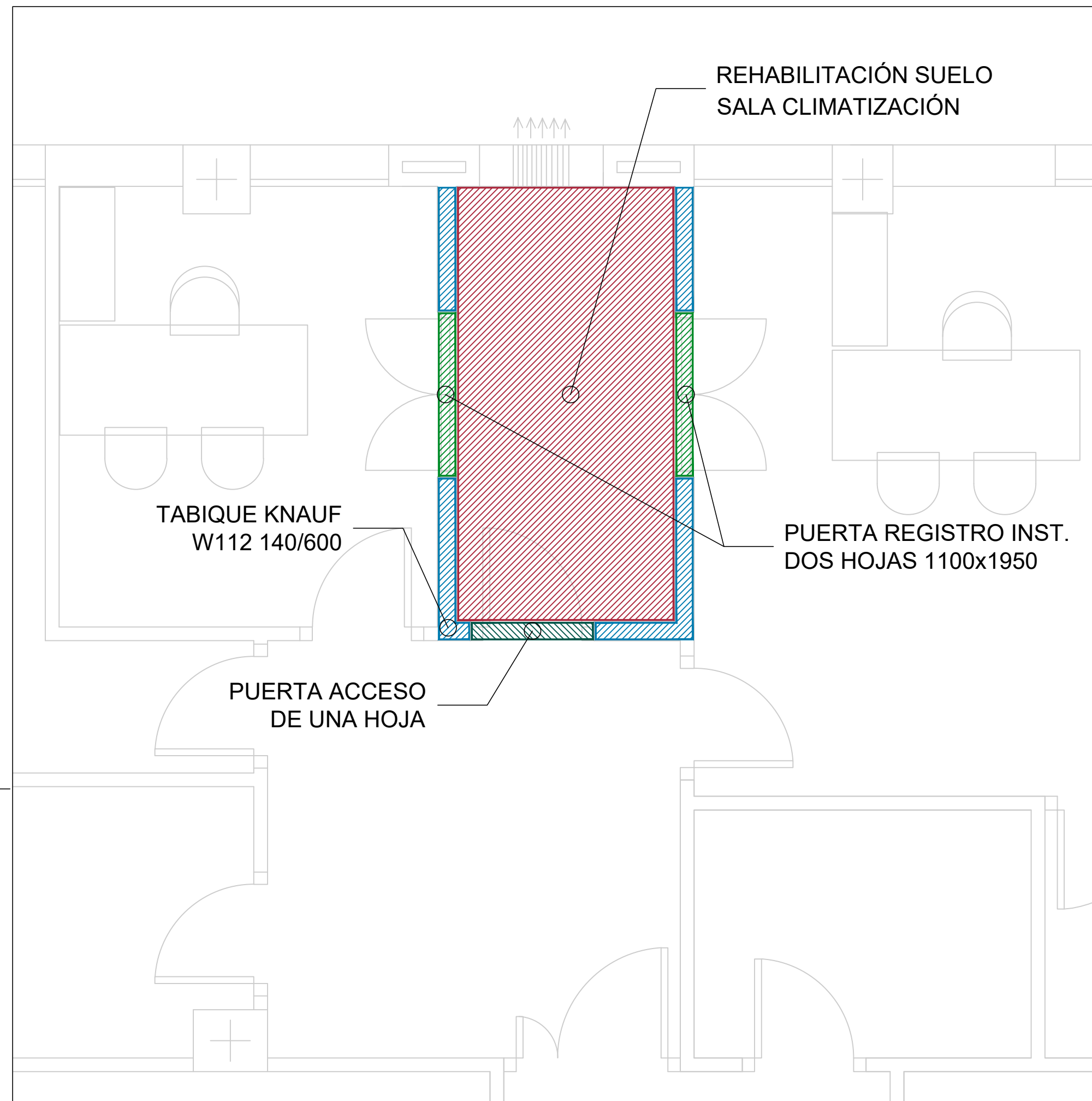
REFORMA SALA CLIMATIZACIÓN (ZONA 2)
