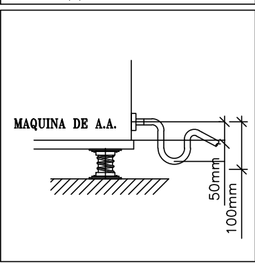
DETALLE (d) : SIFÓN EN DESAGUE
