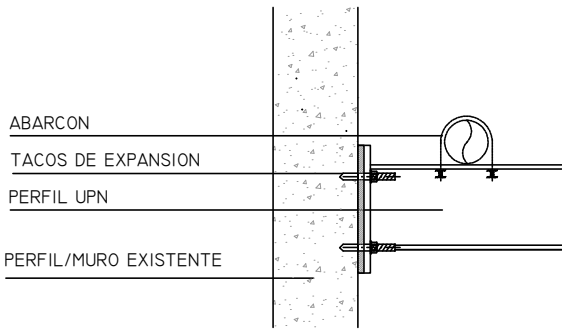
DETALLE 1:
