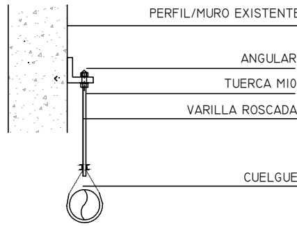
DETALLE 3:
