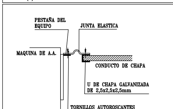
DETALLE (b) : SUBJECCION DE CONDUCTOS
