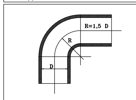
DETALLE (c) : RADIO TÍPICO DE CONDUCTOS
