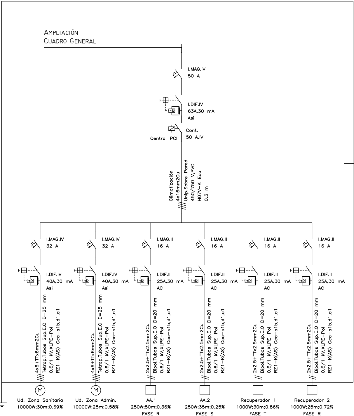
Cuadro General de Mando y Protección
