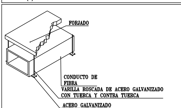
DETALLE (a) : SUBJECCION DE CONDUCTOS
