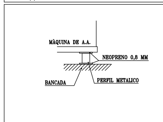
DETALLE (e) : MUELLE ANTIVIBRATORIO
