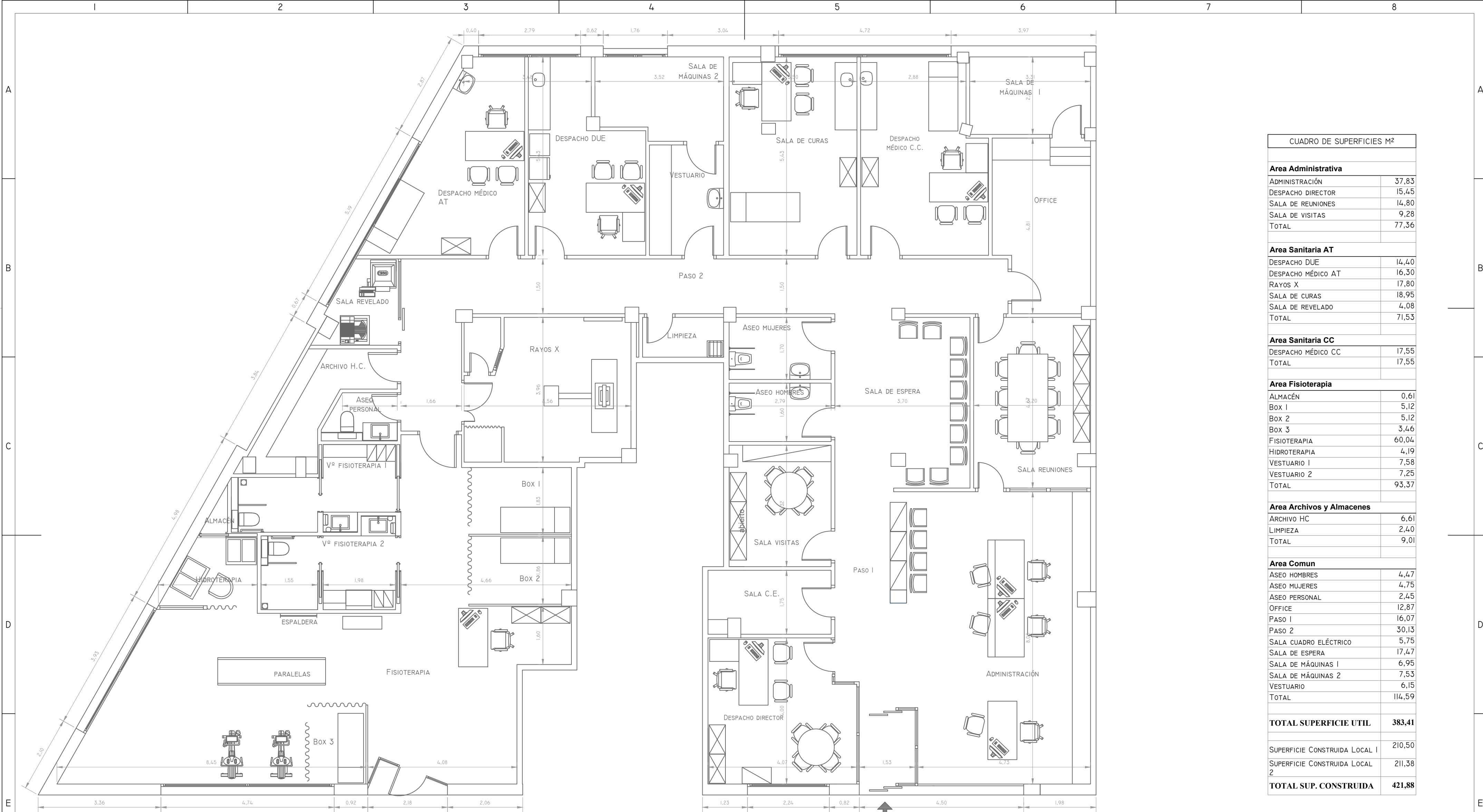
PLANTA BAJA
